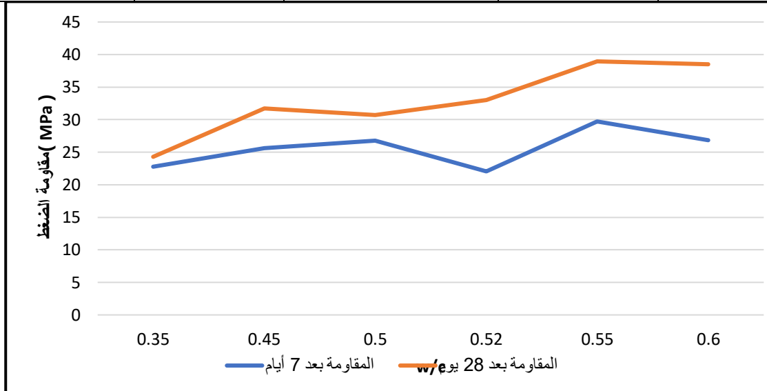
شكل (3) مقاومة الضغط عند استخدام الملدن العادى
