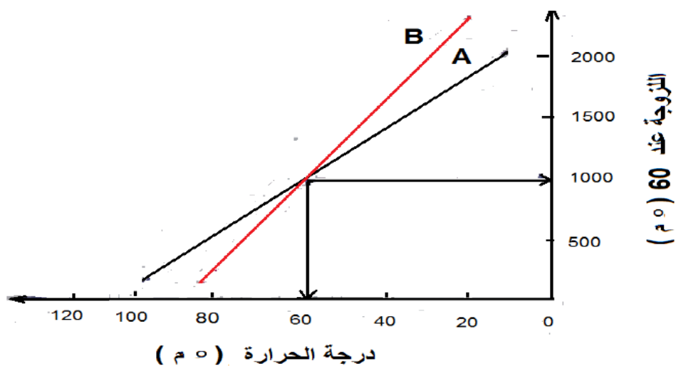
شكل رقم (1): مقارنة بيانية لمادتين اسفلتيتين رابطتين تستوفيان مواصفات تصنيف اللزوجة
