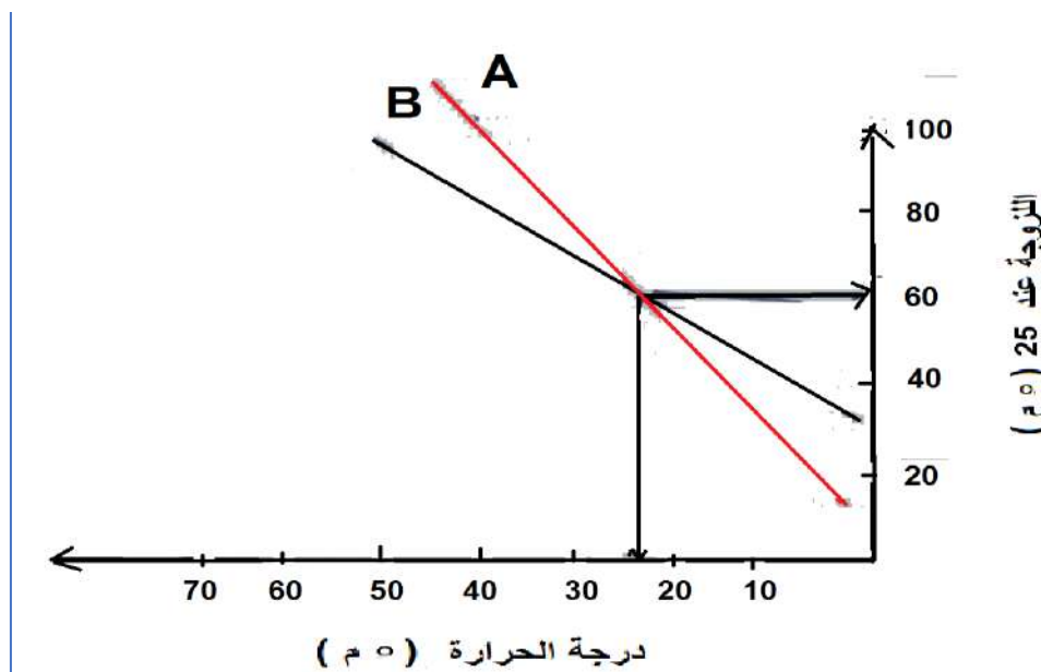
شكل رقم (2) مقارنة بيانية لمادتين رابطتين تستوفيان مواصفات تصنيف الغرز تحتاج الى تغيير الكتابة على المحور الصادي من لزوجة الى (الغرز عند 25) 3 - نظام الاداء لتصنيف المادة الرابطة الاسفلتية
