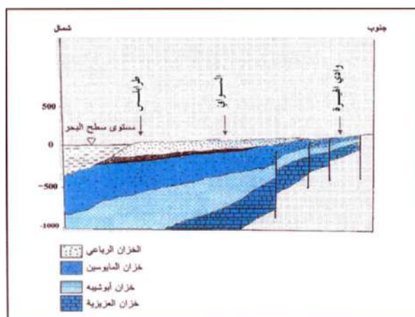
شكل (2) قطاع هيدرولوجي للخزانات الجوفية بالمنطقة (4)
